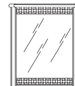
Mirror Intreccio Specchiera intreccio W. 84 H. 110 095SPE.01NO Vol. 0,10 mc - Box 1 - kg 17
