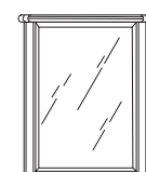
Mirror Rombi Specchiera Rombi W. 84 H. 100 095SPE.02NO Vol. 0,10 mc - Box 1 - kg 10,80
